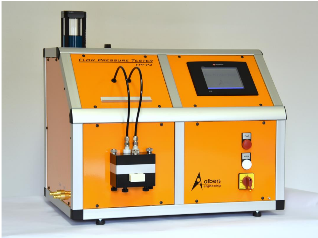
Flow Pressure Tester FPT-P2 (Version mit 2 Prüfplätzen)
